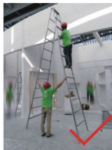
正确的登高作业：2人，1人登高、1人看护，不得站立在梯子最顶层作业，不得使用劣质人字梯。
