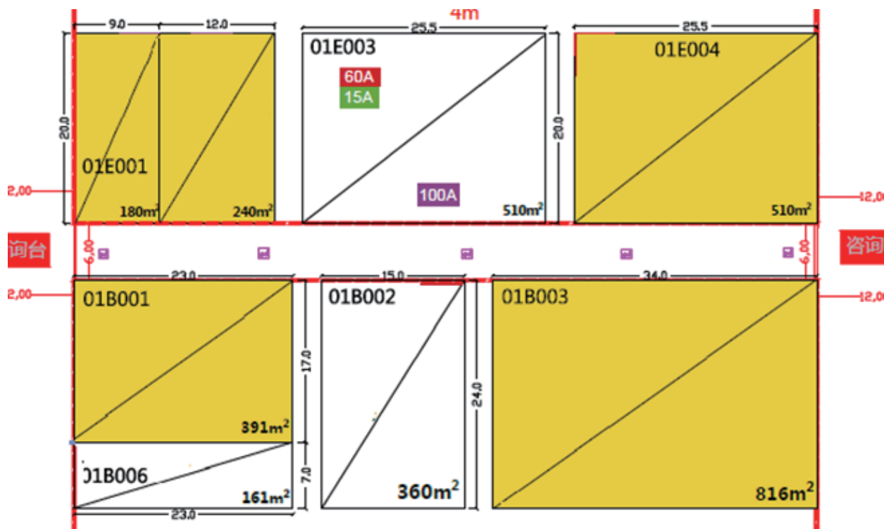
*电箱位置图示例图(必须提交)
